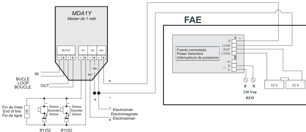
Esquema de conexión FAE03/05 con módulo de relés
