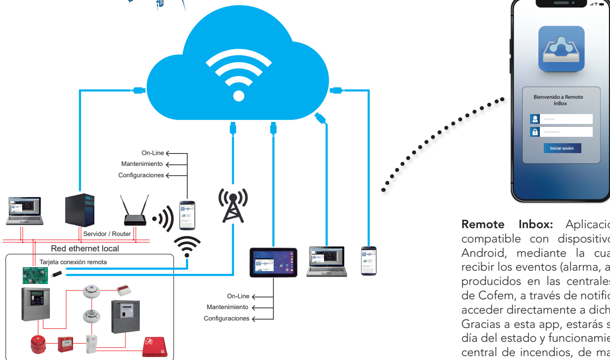
Distribución de elementos dentro de una instalación
