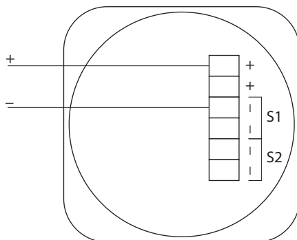
Esquema para SIR24SC
