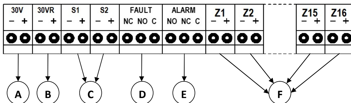
Figura 4: Esquema de los conectores de la central Silver.
